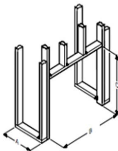
Rohbau Rahmenmaße
